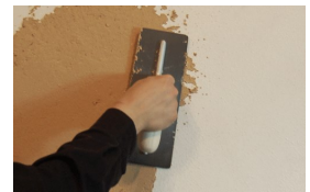
Levitys teräslastalla
